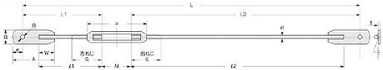
■寸法図
